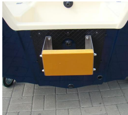
pantograf stały INOX ze wzmoc. i montażem (do silnika z krótką stopą max.10 KM)
